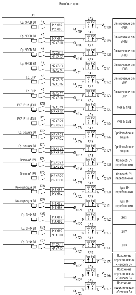
Рисунок В.4 – Схема электрическая принципиальная (часть 4)
